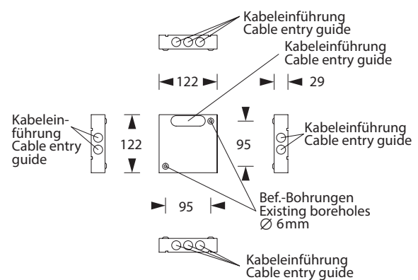
Hinterbaukasten/Back box
